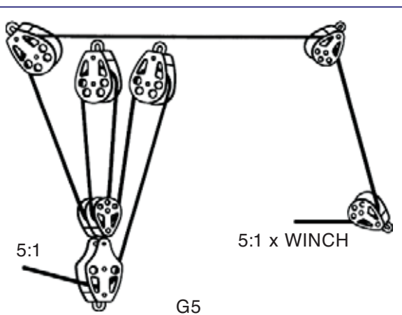
DOPPELTES SYSTEM
