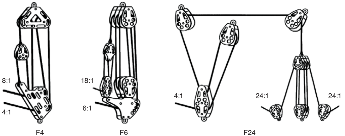
DOPPELTE GROBSCHOTSYSTEME
