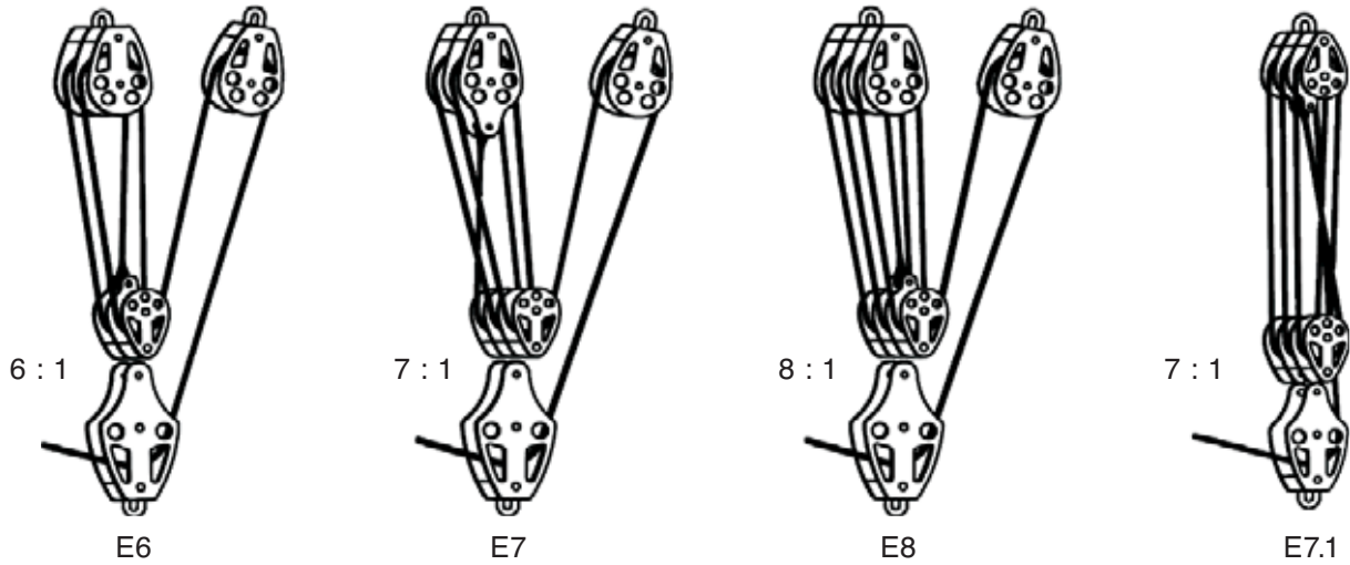
EINFACHE GROBSCHOTSYSTEME
